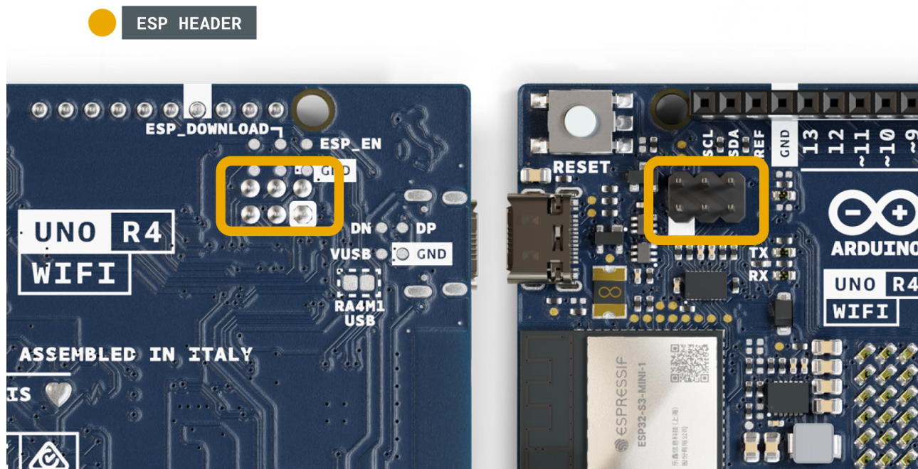
ESP header.
